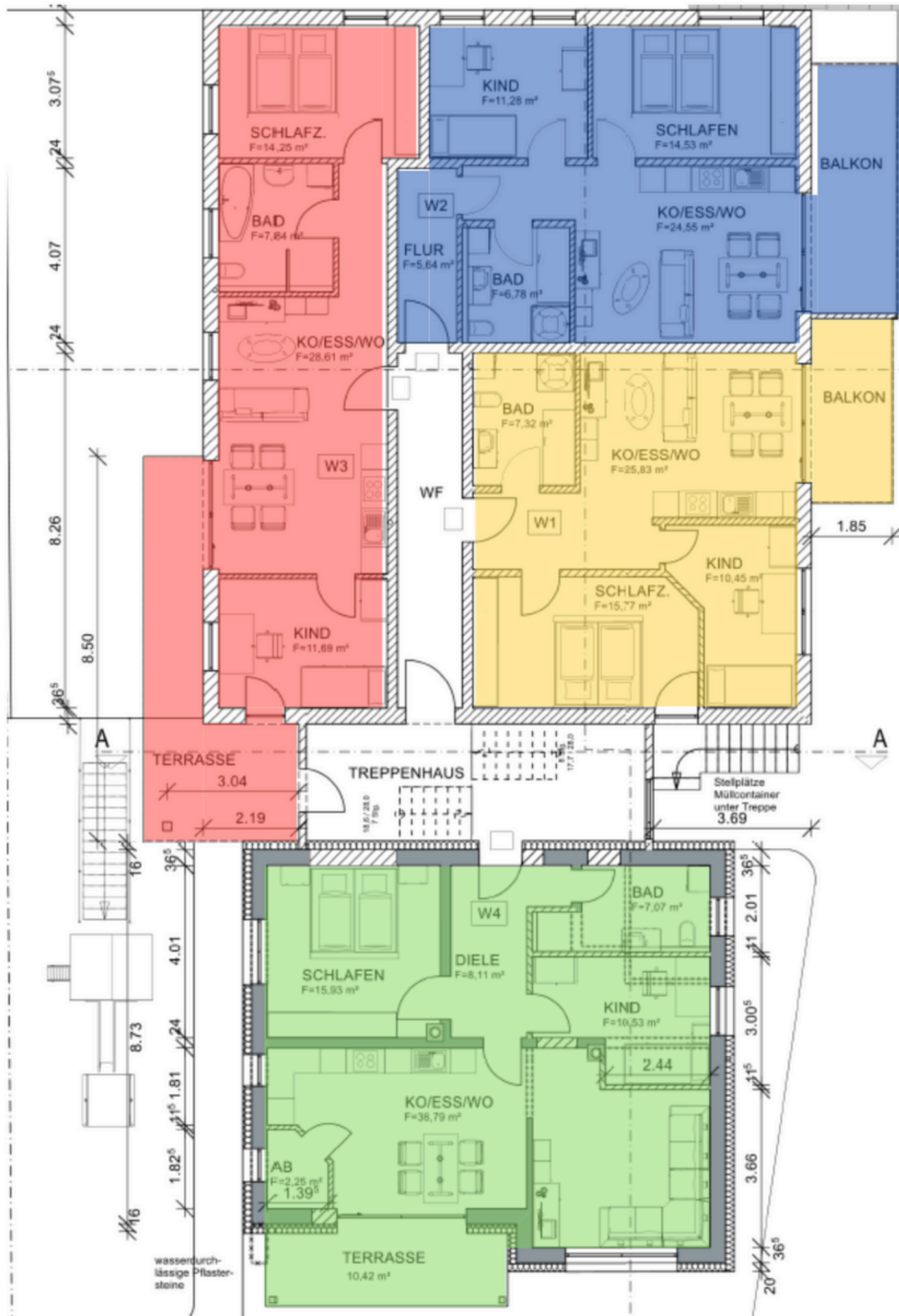
Erdgeschoss
