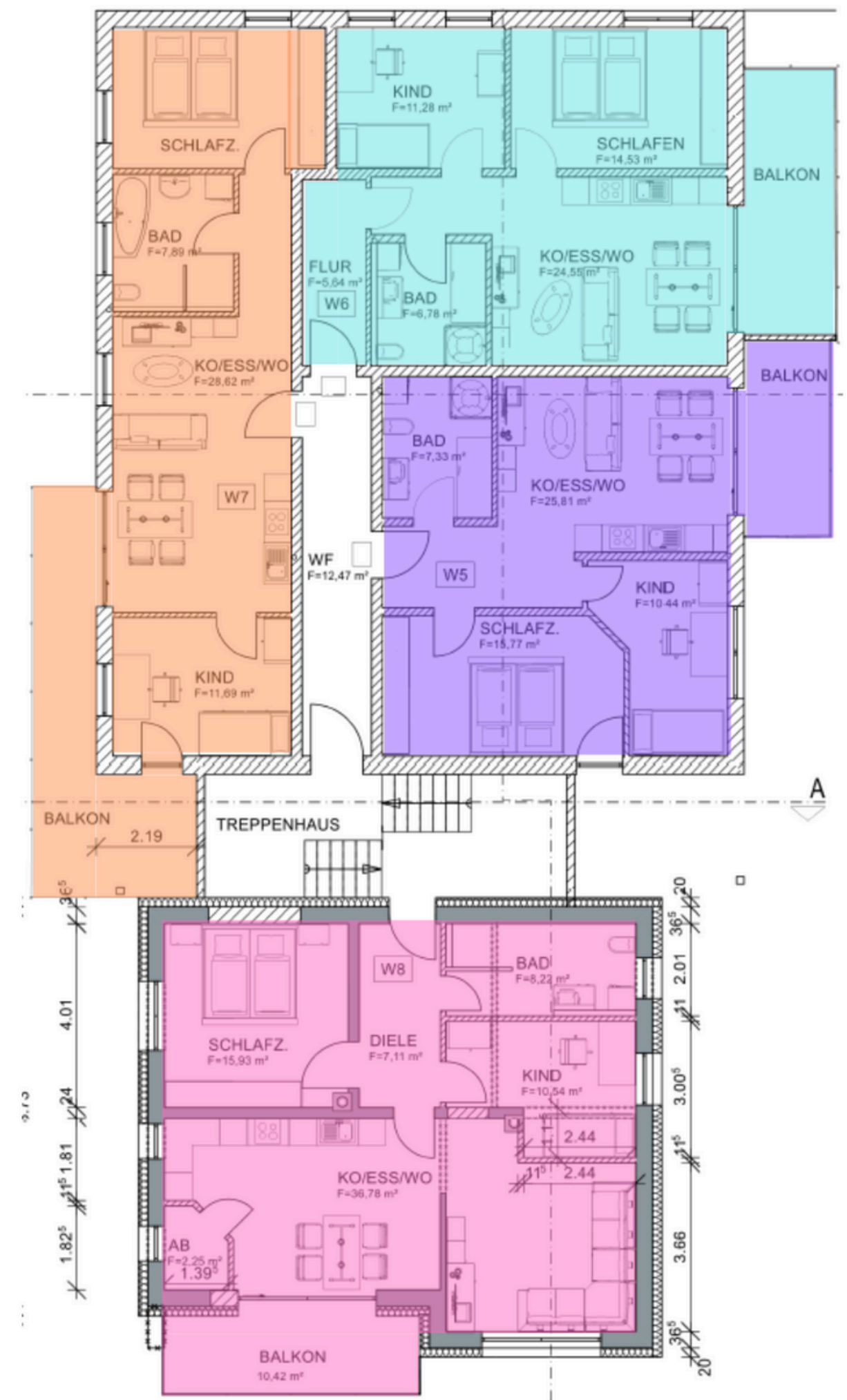
Obergeschoss
